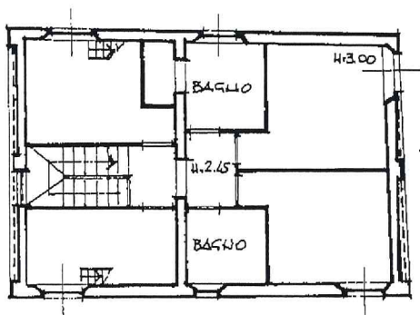
- PIANO PRIMO -
